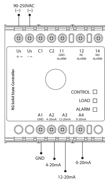
Input type 'I', external AC supply RGC..I..AM, AFM RGC..I..AP, AFP
