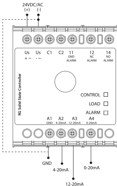
Input type 'I', external DC supply RGC..I..DM, DFM RGC..I..DP, DFP
